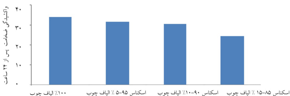
شکل ۱۶. اثر درصد اختلاط بر واکنشیدگی ضخامت پس از ۲۴ ساعت غوطه‌وری در آب
