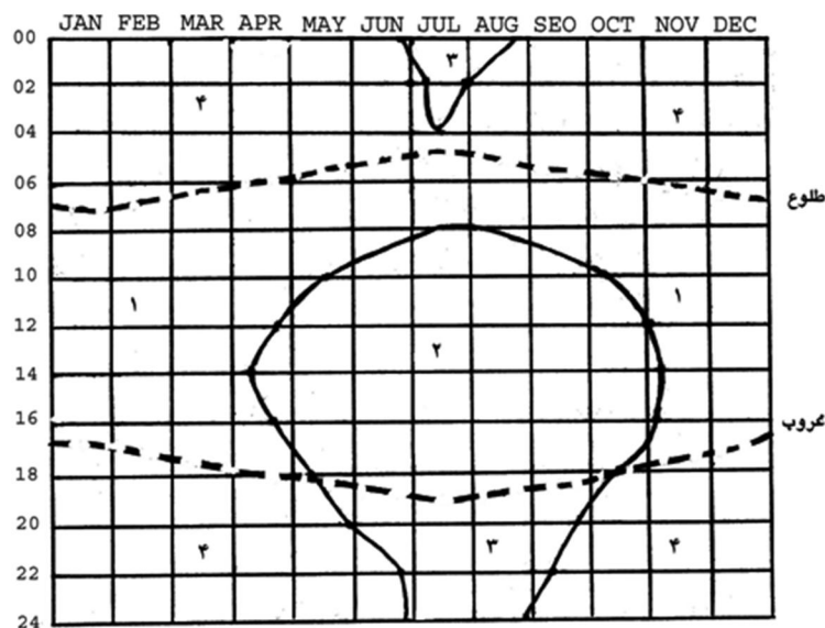
(۱) محدوده نیاز به آفتاب (۲) مواقع گرم شب (۲) محدوده نیاز به سایه (۴) مواقع سرد شب نگاره شماره (۵): تقویم نیاز سایه و آفتاب خرم آباد مأخذ: نگارنده
