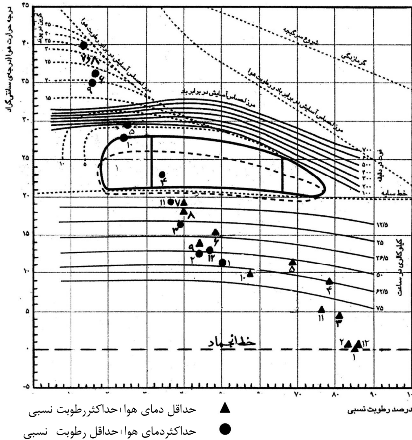
نگاره شماره (۳): جدول بیوکلیماتیک خرم‌آباد
