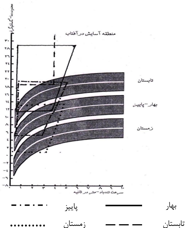
نگاره شماره (۶): معیار راحتی بافت خرم‌آباد (در آفتاب)
