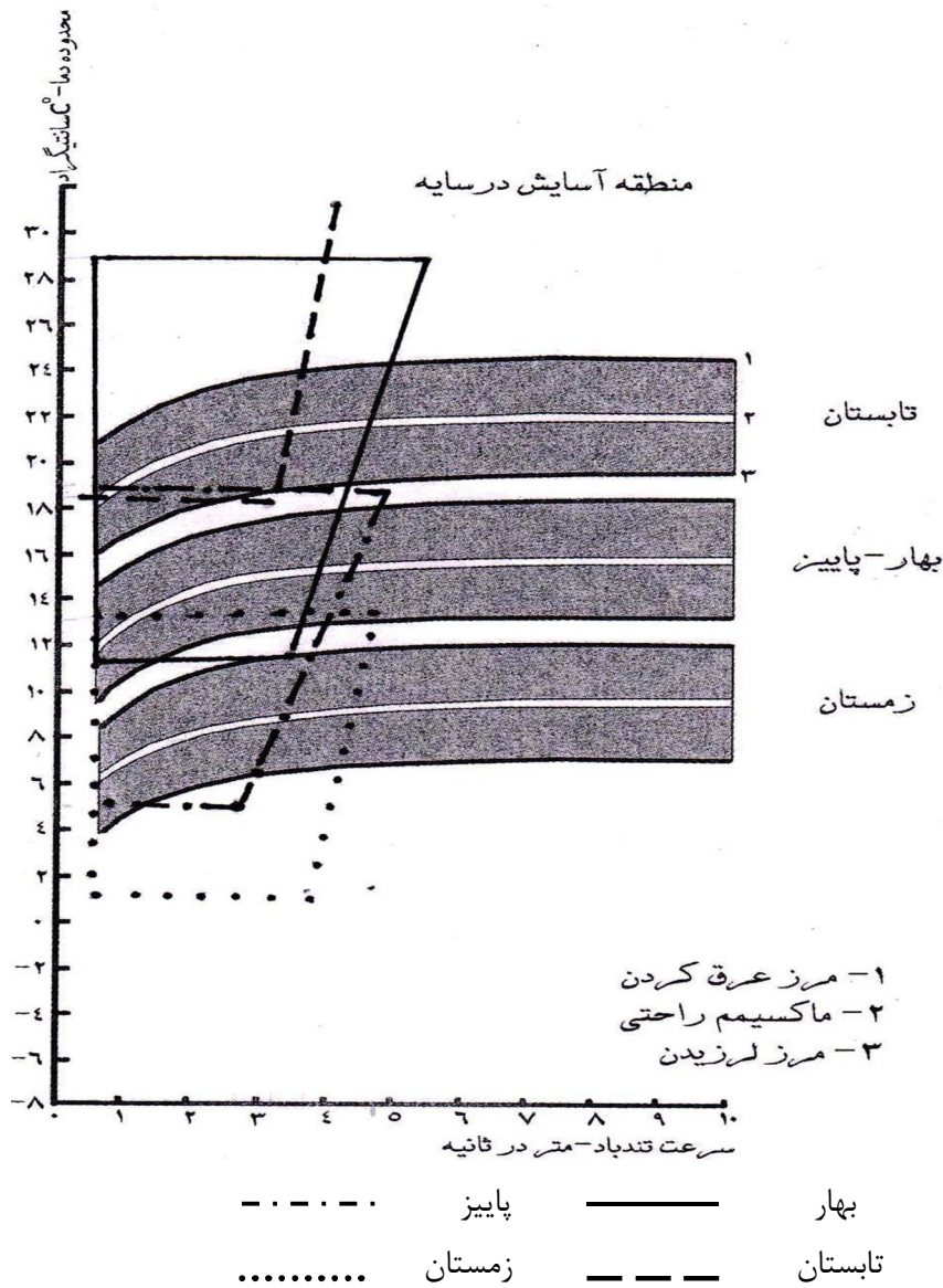
نگاره شماره (۷): معیار راحتی بافت خرم‌آباد (در سایه)
