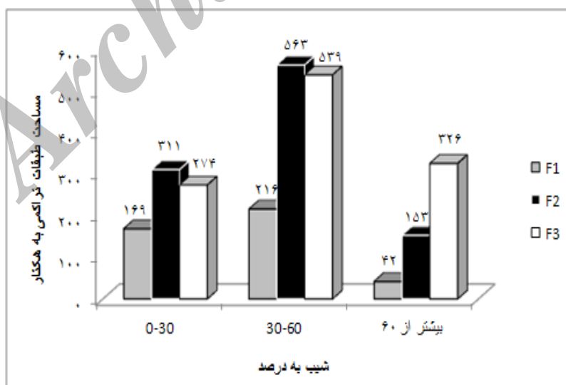
شکل ۲- مساحت طبقات تراکمی در شیب های مختلف در سال ۱۳۳۴
