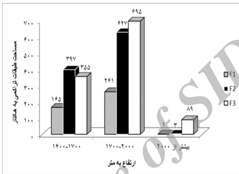
شکل ۶- مساحت طبقات تراکمی در ارتفاع های مختلف در سال ۱۳۳۴
