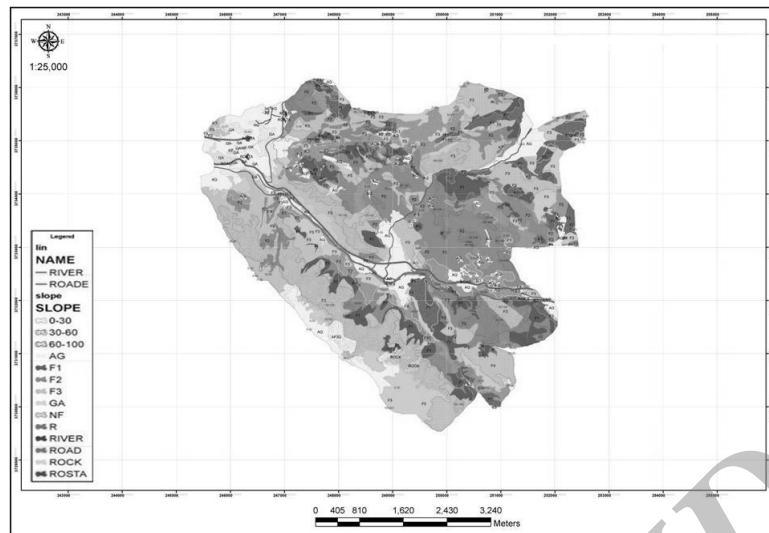
شکل ۳- پوشش منطقه در شیبهای مختلف با استفاده از عکسهای هوایی سال ۱۳۳۴
