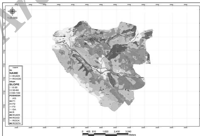
شکل ۵- پوشش منطقه در شیب های مختلف با استفاده از عکسهای هوایی سال ۱۳۷۶
