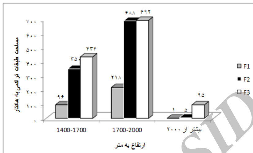
شکل ۸- مساحت طبقات تراکمی در ارتفاعهای مختلف در سال ۱۳۷۶
