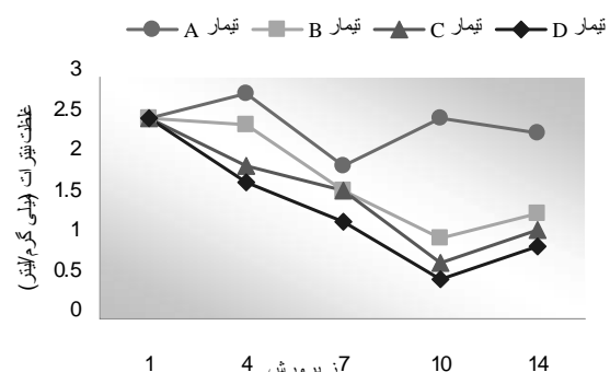
شکل ۵- غلظت باقیمانده نیتريت (NO 3 ) پساب در طول آزمایش
