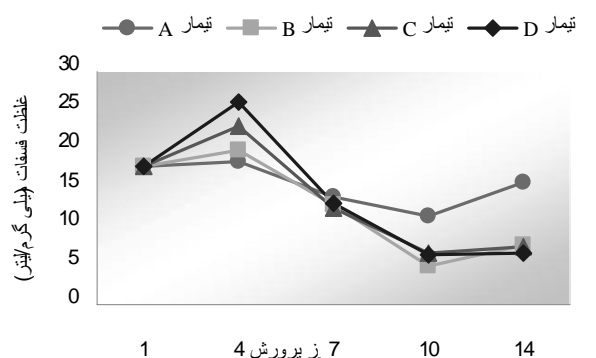
شکل ۷- غلظت باقیمانده فسفات (PO 4 ) پساب در طول آزمایش
