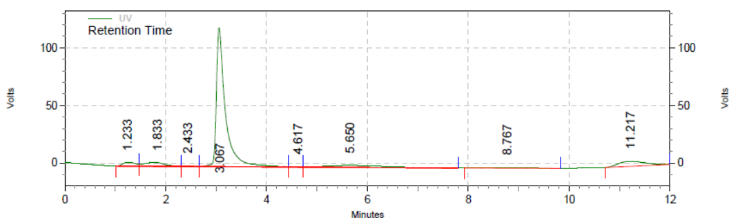
نمودار (۱) - کروماتوگرام طیف استاندارد انروفلوکسازین
