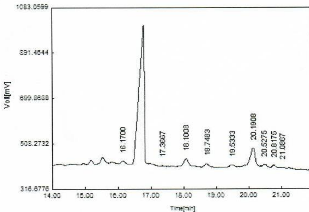
نمودار (۳) - کروماتوگرام ترکیبات استرولی روغن کنجد
