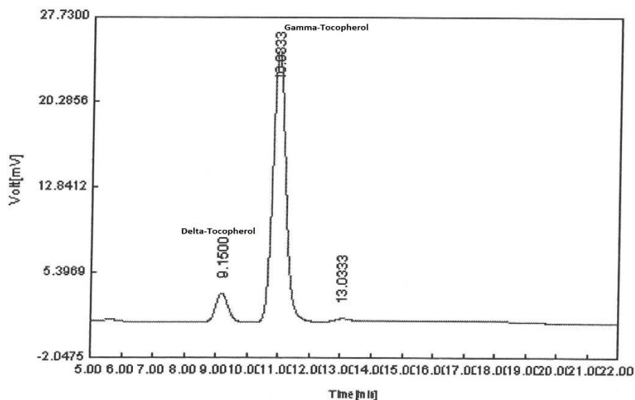
نمودار (۲) - کروماتوگرام ترکیبات توکوفرولی روغن کنجد
