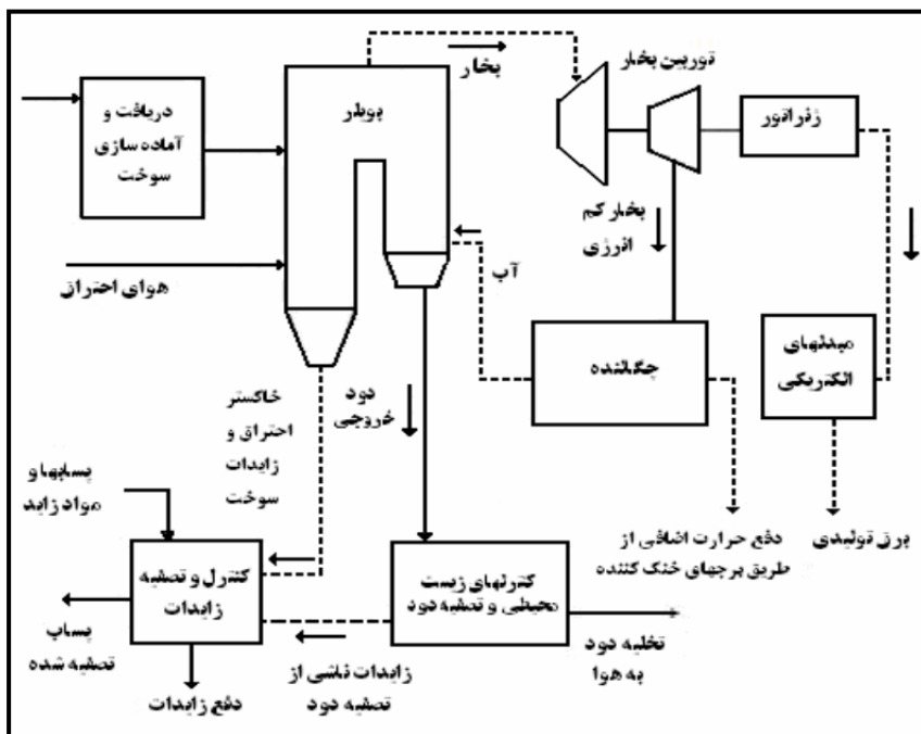
شکل ۱. اجزای اساسی یک نیروگاه حرارتی با توربین بخار (۳)
