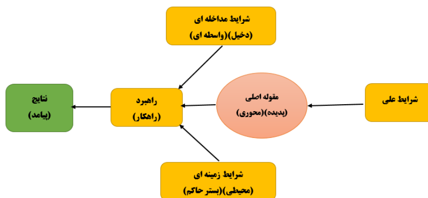
شکل ۱- مدل پارادایمی
