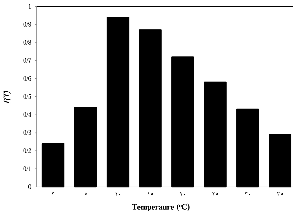
شکل ۲- مقادیر f(T) برای دماهای ثابت مختلف بر اساس مدل دو تکه‌ای
