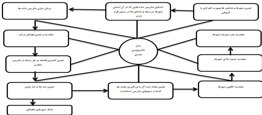
شکل (۲): فرایند انجام تاکسونومی عددی
