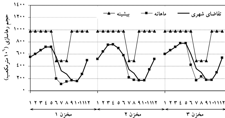
شکل ۵. تغییرات ماهانه حجم تقاضای شهری و رهایسازی از مخازن مختلف در حالت SRSO با هدف تأمین تقاضای شهری
