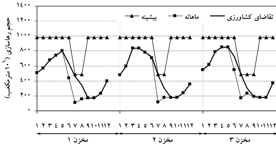
شکل ۴. تغییرات ماهانه حجم تقاضای کشاورزی و رهایسازی از مخازن مختلف در حالت SRSO با هدف تأمین تقاضای کشاورزی
