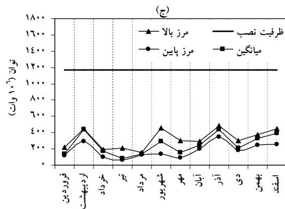
شکل ۹. نتایج تحلیل برای مخزن ۱ در حالت SRMO: (الف) مجموعه نقاط پرتو برای تابع هدف‌های مورد بررسی، (ب) محدوده تغییرات ماهانه حجم تقاضا و رها سازی کشاورزی، (پ) محدوده تغییرات ماهانه حجم تقاضا و رها سازی شهری، (ت) محدوده تغییرات ماهانه حجم تقاضا و رها سازی صنعتی، (ث) محدوده تغییرات ماهانه حجم رها سازی تفریحات و کنترل سیلاب و (ج) محدوده تغییرات ماهانه توان تولیدی
