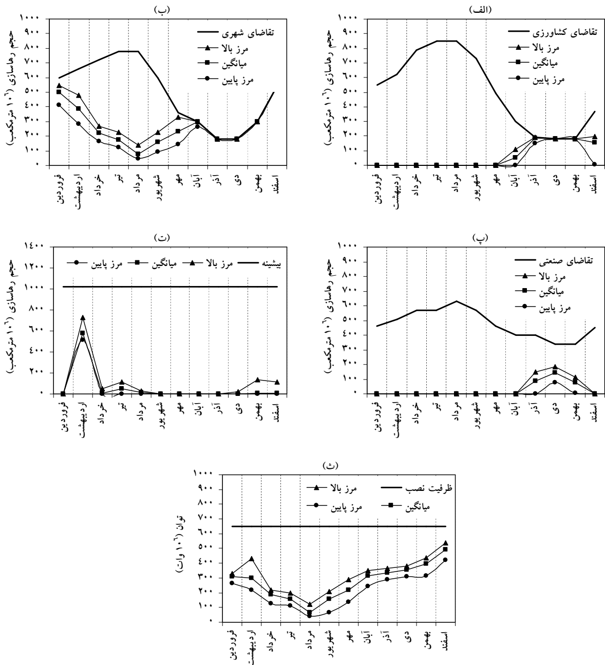
شکل ۲۲. نتایج تحلیل برای مخزن ۳ در حالت MRMO: (الف) محدوده تغییرات ماهانه حجم تقاضا و رهاسازی کشاورزی، (ب) محدوده تغییرات ماهانه حجم تقاضا و رهاسازی شهری، (پ) محدوده تغییرات ماهانه حجم تقاضا و رهاسازی صنعتی، (ت) محدوده تغییرات ماهانه حجم رهاسازی تفریحات و کنترل سیلاب و (ث) محدوده تغییرات ماهانه توان تولیدی
