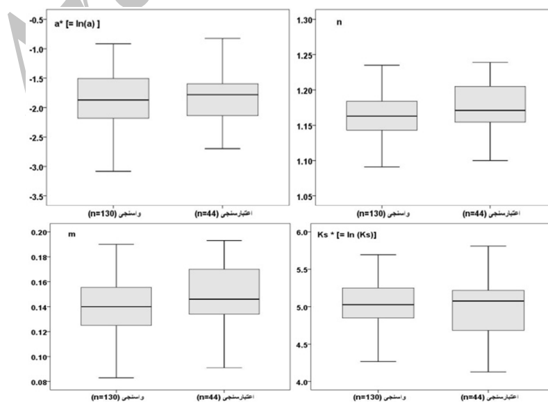
شکل ۲. پلات‌های جعبه‌ای توزیع و گستره کمی پارامترهای هیدرولیکی خاک به ازای داده‌های واسنجی و اعتبارسنجی
