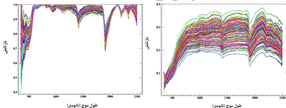
شکل ۳. منحنی‌های خام بازتاب طیفی (راست) و منحنی‌های حذف پیوستار بازتاب طیفی (چپ) خاک‌های مورد مطالعه
