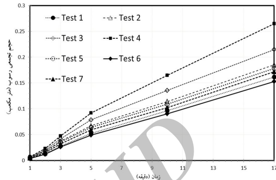
شکل ۹. حجم تجمعی رسوب
