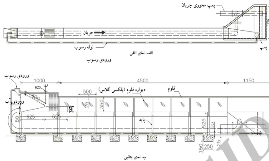
شکل ۱. سامانه آزمایشگاهی
