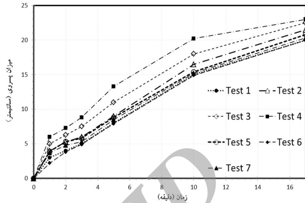
شکل ۵. میزان پس روی پیشانی پرتگاه نسبت به زمان
