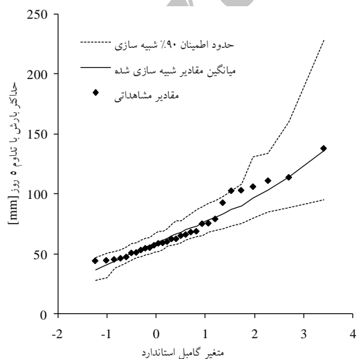
شکل ۲. ارزیابی عملکرد مدل NSRP در بازتولید ویژگی‌های بارش مشاهده‌ای. ویژگی‌های آماری بارش روزانه و توزیع بارش‌های حدی مشاهده‌ای کرمانشاه با حدود ۹۰٪ ویژگی‌های متناظر ۱۰۰ سری ۳۰ ساله بارش شبیه‌سازی شده توسط مدل NSRP مقایسه شده است.
