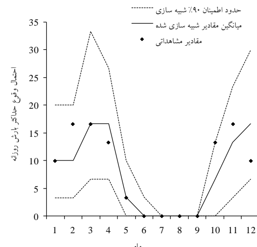
شکل ۲. ارزیابی عملکرد مدل NSRP در بازتولید ویژگی‌های بارش مشاهده‌ای. ویژگی‌های آماری بارش روزانه و توزیع بارش‌های حدی مشاهده‌ای کرمانشاه با حدود ۹۰٪ ویژگی‌های متناظر ۱۰۰ سری ۳۰ ساله بارش شبیه‌سازی شده توسط مدل NSRP مقایسه شده است.
