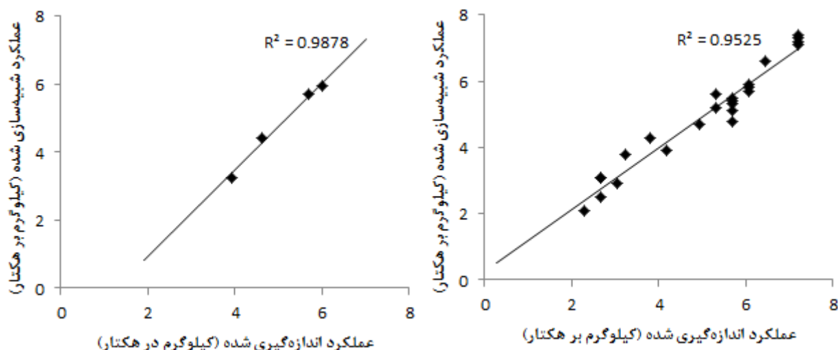
شکل ۵. برازش مقادیر اندازه‌گیری شده و شبیه‌سازی شده عملکرد زعفران در دو مرحله واسنجی (راست) و صحت‌سنجی (چپ) با استفاده از مدل AquaCrop
