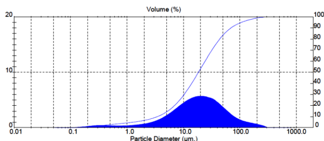
شکل ۵. منحنی درصد کوچکتر از هر اندازه تجمعی و منحنی فراوانی برای مواد فیلتر شده توسط فیلتر توری شاهد
