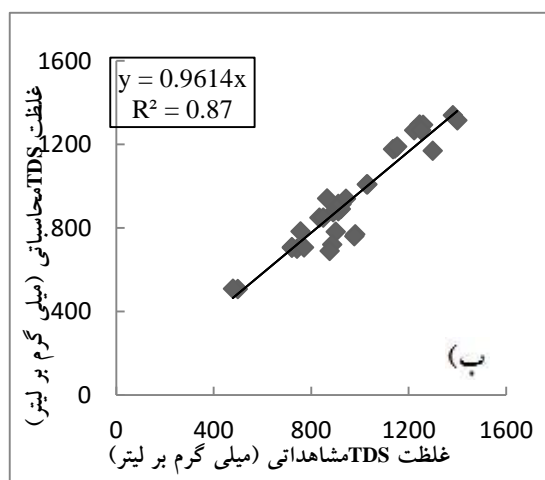
شکل ۷. نتایج الف) واسنجی مدل کیفی در شرایط غیرماندگار، ب) صحت‌سنجی مدل کیفی
