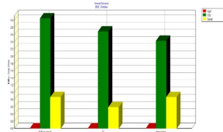
شکل ۱۲. حساسیت بالای سناریو تصفیه‌خانه T1 جهت تأمین مصارف کشاورزی در تابع هدف، تخلیه کمتر آبخوان در سال
