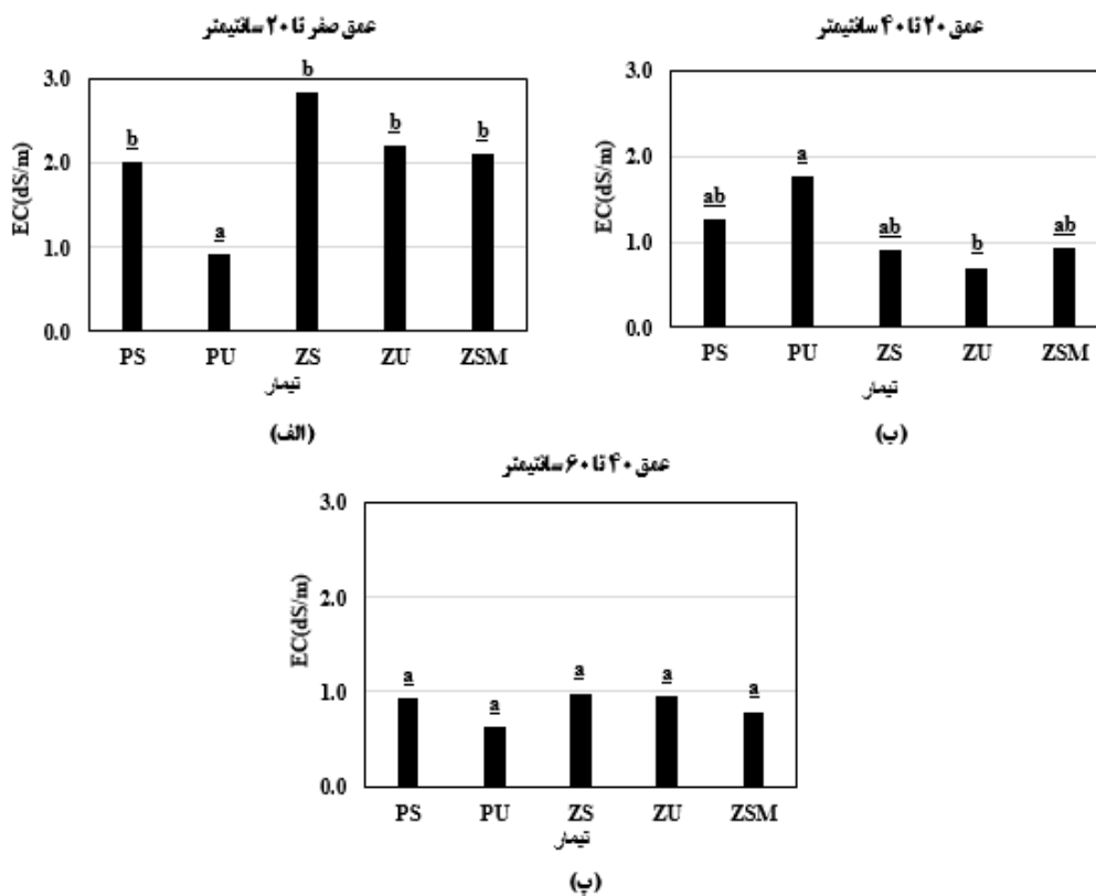
شکل ۶. مقایسه میانگین‌های شوری در هر پنج تیمار در اعماق ۲۰-۰ (الف)، ۴۰-۲۰ (ب) و ۶۰-۴۰ (پ) و در فاصله ۱۵ سانتی‌متر از گسیلنده
