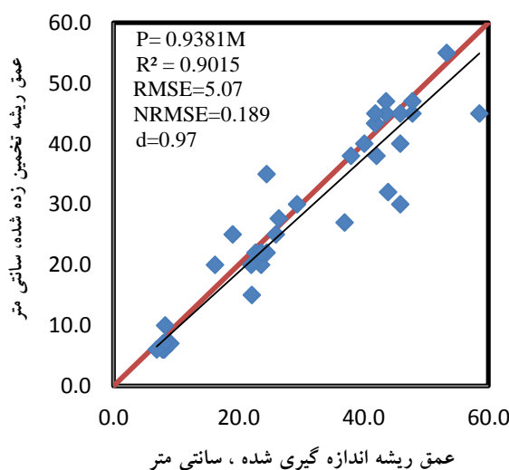
شکل ۷. مقایسه نتایج معادلات تعیین عمق ریشه و مقادیر اندازه‌گیری شده نسبت به خط یک‌به‌یک
