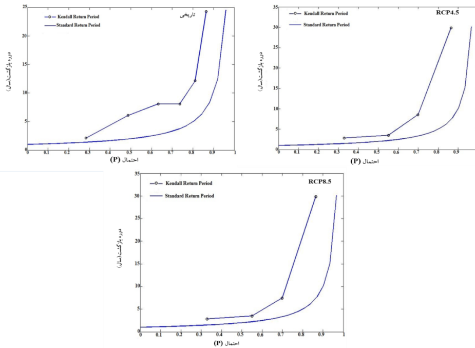
شکل ۹. دوره بازگشت کندال، T_p بر اساس تابع توزیع کندال تجربی و دوره بازگشت استاندارد، T'_{DS} بر اساس توابع مفصل جوئی برای داده‌های تاریخی ایستگاه ارومیه و داده‌های پیش‌بینی شده تحت سناریوهای مورد مطالعه در افق نزدیک (۲۰۳۰-۲۰۱۱)
