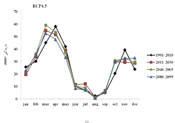
شکل ۳. نمودار بارش مشاهداتی و پیش‌بینی شده ایستگاه ارومیه برای داده‌های تاریخی سه سناریو RCP4.5 و RCP8.5 برای سه افق نزدیک، میانی و دور
