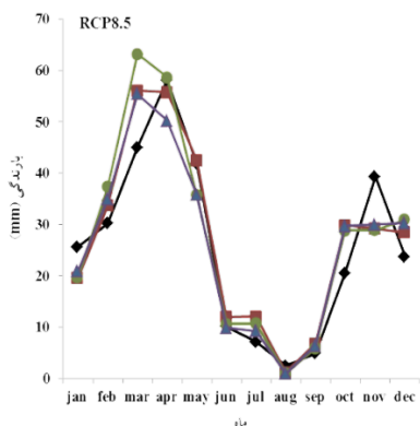
شکل ۳. نمودار بارش مشاهداتی و پیش‌بینی شده ایستگاه ارومیه برای داده‌های تاریخی سه سناریو RCP4.5 و RCP8.5 برای سه افق نزدیک، میانی و دور
