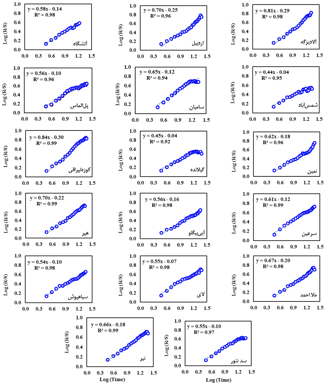
شکل ۲. دامنه مقیاس‌بندی شده حداکثر بارش سالانه در ایستگاه‌های باران‌سنجی منتخب استان اردبیل
