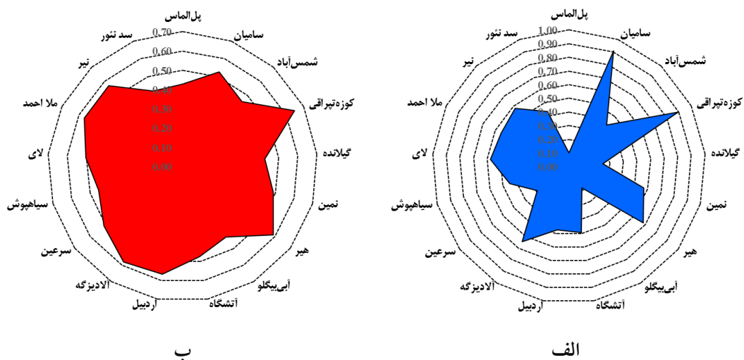
شکل ۵: تغییرات مقادیر تجزیه و تحلیل پراکندگی (الف) و ریسک EDEC (ب) در ایستگاه‌های باران‌سنجی منتخب استان اردبیل
