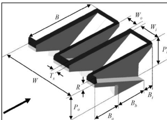
شکل ۱. پارامترهای اصلی سرریز کلید پیانویی
