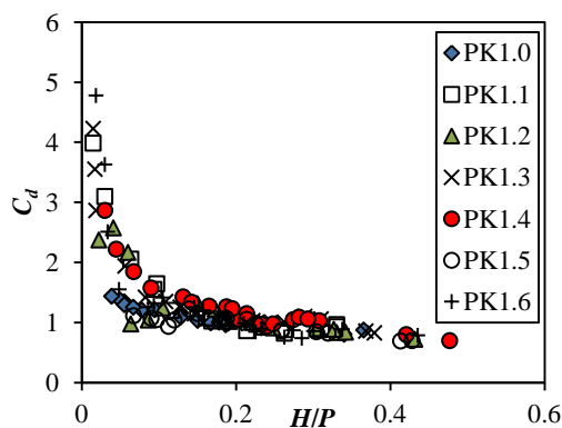
شکل ۶. تغییرات ضریب تخلیه (Cd) در برابر نسبت H/P در انواع سرریزهای کلید پیانویی
