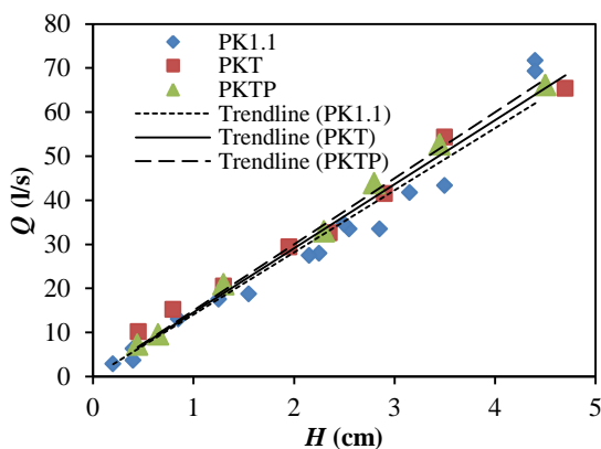
شکل ۸. تغییرات دبی ( Q ) در برابر ارتفاع ( H ) در سرریزهای PKTP و PKT، PK1.1
