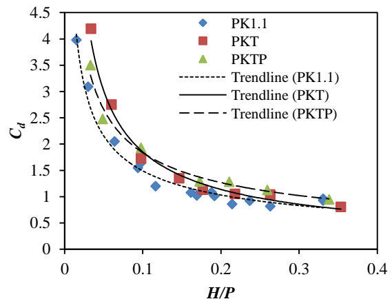
شکل ۹. تغییرات ضریب تخلیه ( C_d ) در برابر نسبت H/P در سرریزهای PK1.1 ، PKT و PKTP
