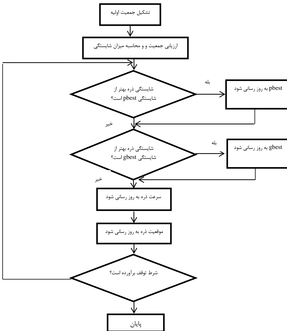
شکل ۲ - فلوجارت الگوریتم بهینه‌سازی انبوه ذرات مأخذ: بهمنی و همکاران [۲۰]
