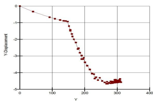
شکل 8: جابجایی قائم در ansys و geo studio
