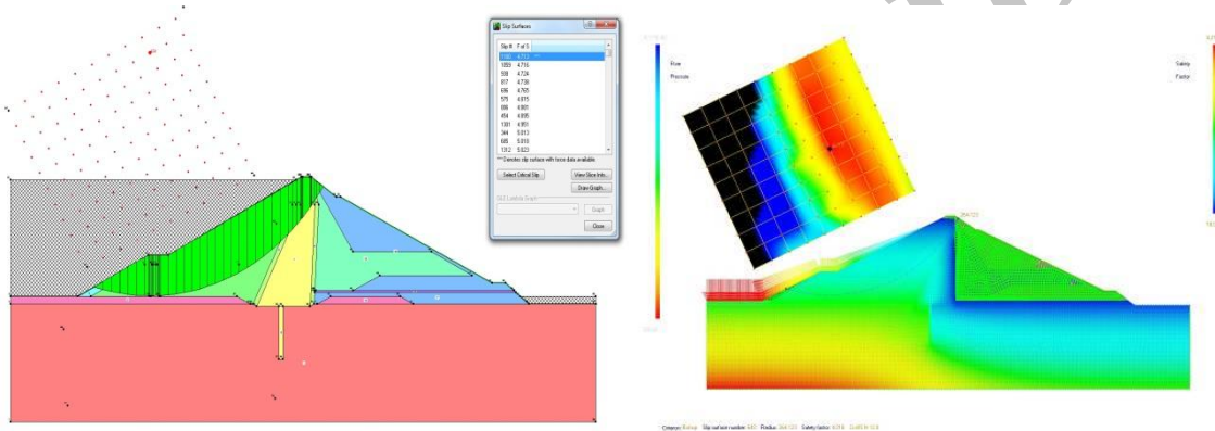
شکل 9: سطح بحرانی به روش بیشاپ در بالا دست (ansys , geostudio)
