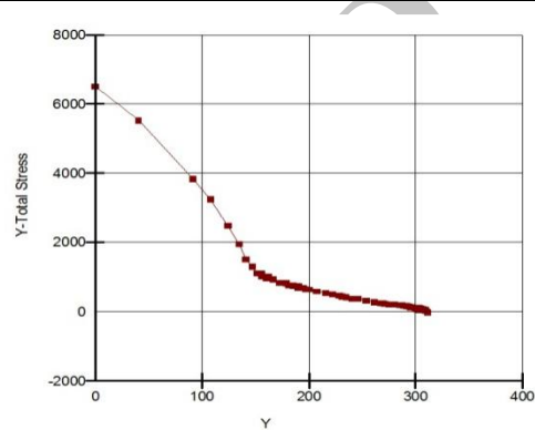
شکل 7: تنش کل قائم در ansys و geo studio
