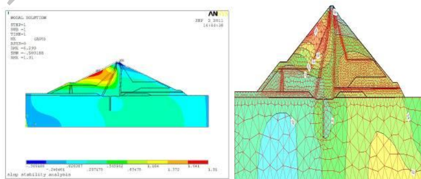
شکل 6: جابجایی در راستای افقی ansys و geo studio
