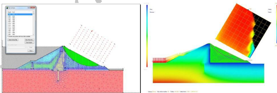
شکل 10: سطح بحرانی به روش بیشاپ در پایین دست (ansys , geo studio)
