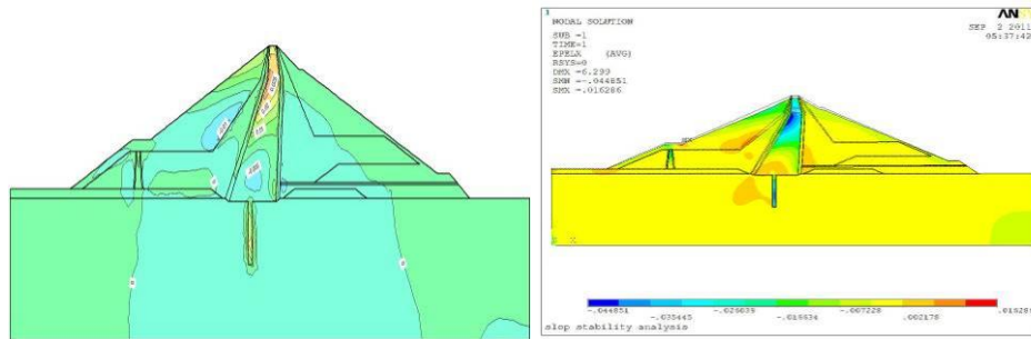
شکل 4: کرنش افقی در Geo Studio و Ansys
