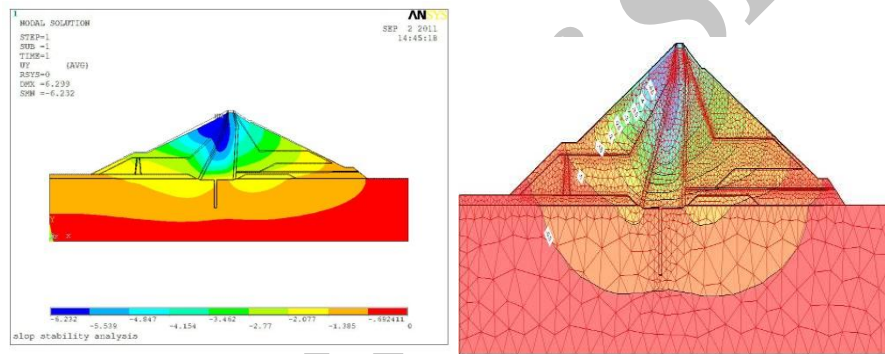
شکل 5: جابجایی در راستای قائم ansys و Geo Studio
