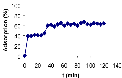
شکل (۱) اثر مدت زمان تماس در میزان جذب سطحی آبی متیلن ([MB]_0=10 \text{ mg/L}; [Nano-TiO_2]=0.1 \text{ g}/250 \text{ mL}; \text{pH}=6; T=25^\circ\text{C})
