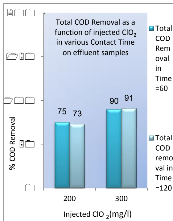
نمودار شماره ۱- نتایج کاهش COD روی نمونه‌های پسب
