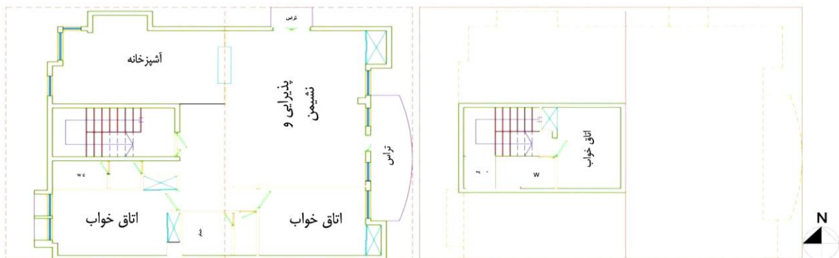
تصویر ۹- پلان طبقه سوم و نیمه طبقه بالای طبقه سوم خانه‌ای در کوچه مختاران
