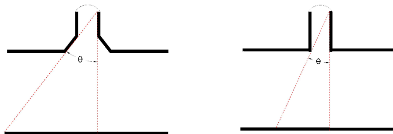
شکل ۵- زوایای انسداد دید در نورگیرهای سقفی (McHugh, Heschong, Manglani, & Dee, 2003).
