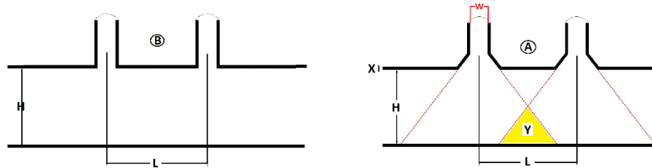
شکل ۲- فاصله دو نوع نورگیر سقفی از یکدیگر (McHugh, Heschong, Manglani, & Dee, 2003).
