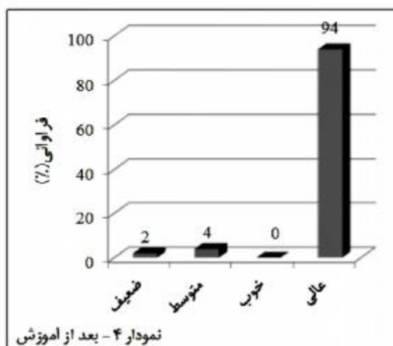
نمودار (۳ و ۴): فراوانی آگاهی دانش آموزان در مقیاس لیکرت در ارتباط با مباحث زیست محیطی قبل و بعد از آموزش
