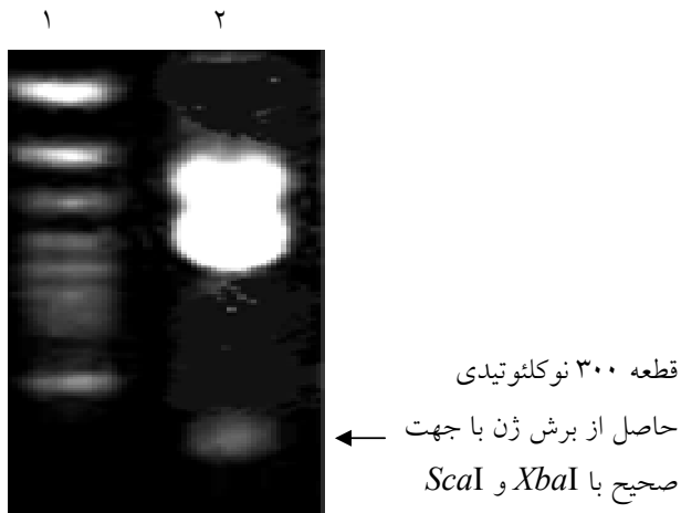
شکل ۱۱- تعیین جهت ژن کلسی توئین با نقشه ژنتیکی. ردیف اول DNA سایز مارکر ۱۰۰ bps، ردیف دوم پلاسمید pPI-Cal بریده شده با ScaI و XbaI
