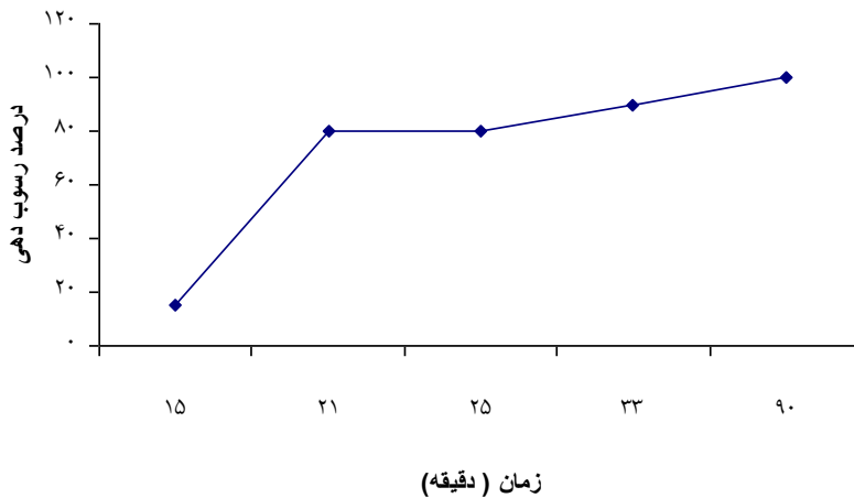
شکل ۲- درصد رسوب دهی میکرو جلیک سندسموس در زمان های مختلف در تیمار دو
