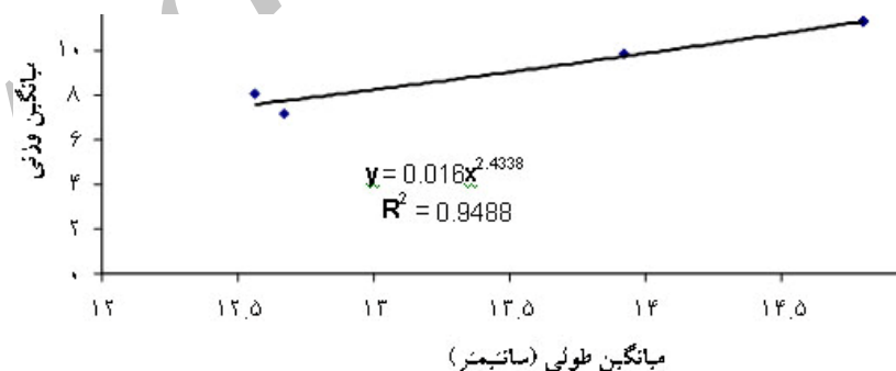
شکل ۸: رابطه میانگین طولی با میانگین وزنی چالباش در سد وشمگیر
