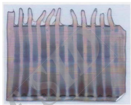
شکل ۱: ژل تهیه شده از استراز ماهی سفید - منطقه دریا
