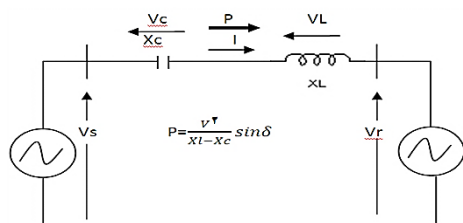
شکل ۱. سیستم ابتدایی دو ماشین با یک خط جبران‌سازی شده با خازن سری [۳].
