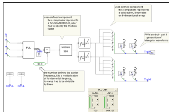
شکل ۱۲. شماتیک قسمت سازنده موج مثلثی PWM (قسمت اول PWM)
