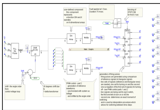
شکل ۱۳. شماتیک قسمت سازنده موج سینوسی PWM (قسمت دوم PWM)
