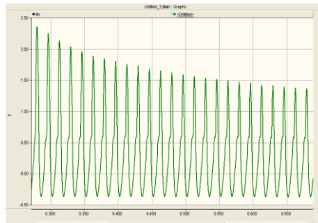
شکل ۸. جریان هجومی بعد از برق‌دار شدن ترانسفورماتور
