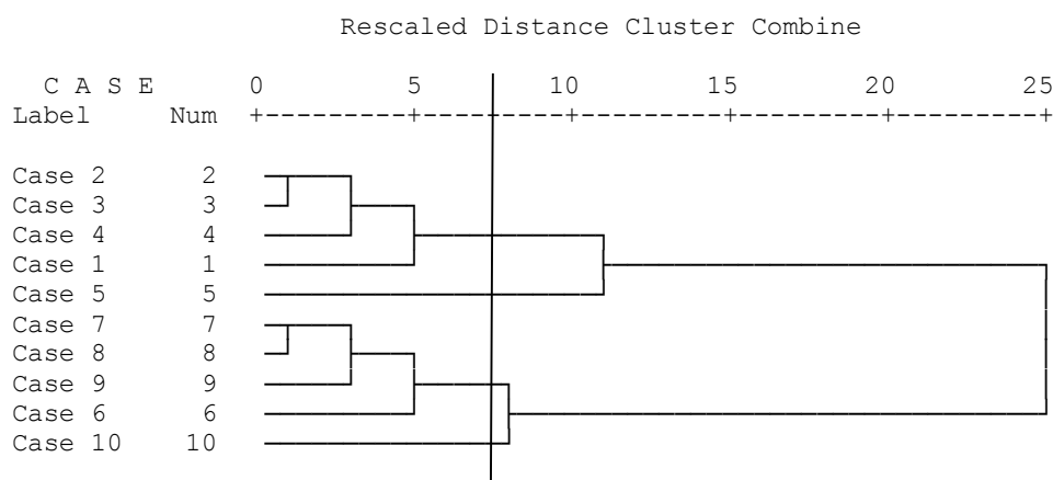
شکل ۲: دندروگرام حاصل از تجزیه خوشه‌ای بر اساس درصد ترکیبات اسانس پونه وحشی
