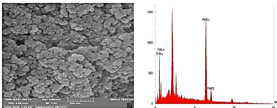
شکل ۵: تصویر میکروسکوپ الکترونی رومیزی (SEM) نانو ذرات اکسید آهن سنتز شده با استفاده از عصاره آبی گیاه خرفه و طیف پراش اشعه ایکس (EDX) مربوط به آن.
