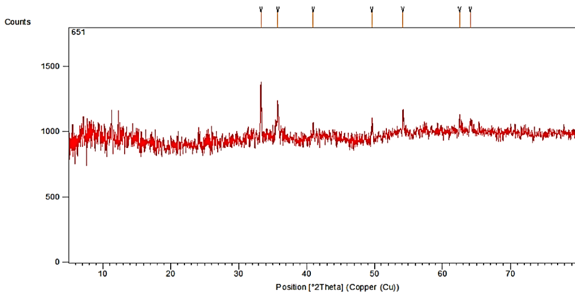
شکل ۴: طیف پراش اشعه ایکس نانو ذرات اکسید آهن سنتز شده با استفاده از عصاره آبی گیاه خرفه
