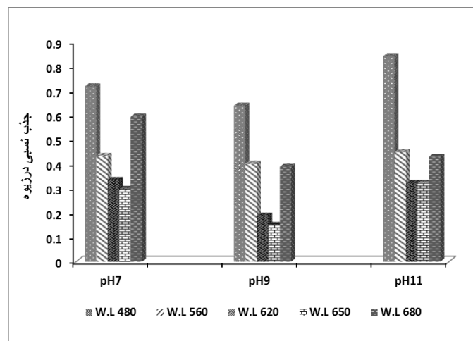
شکل ۳: هیستوگرام مقایسه درزئوه رنگیزه‌ها در سیانوباکتریوم Anabaena sp. FS76 در
