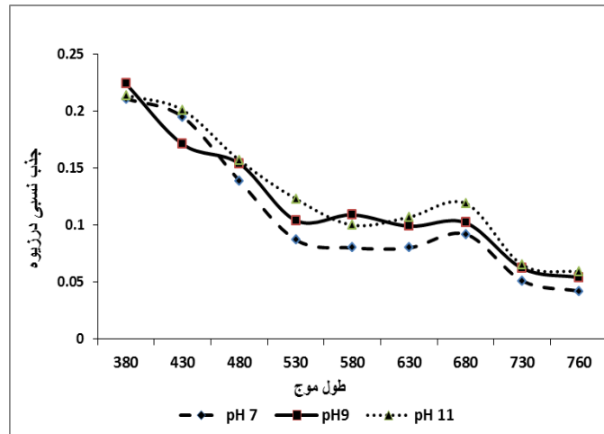
شکل ۲: مقایسه منحنی طیف جذبی درزئوه سیانوباکتریوم Anabaena sp. FS76 در شرایط pH 7,9,11
