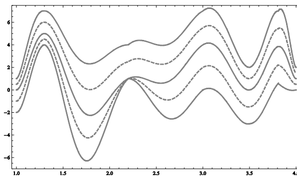
شکل ۳. خطچین‌ها نمایش مجموعه \frac{1}{2} -برش چندجمله‌ای درونیاب هرمیت فازی و خطوط توپر نمایش تکیه‌گاه و هسته چندجمله‌ای درونیاب می‌باشند.
