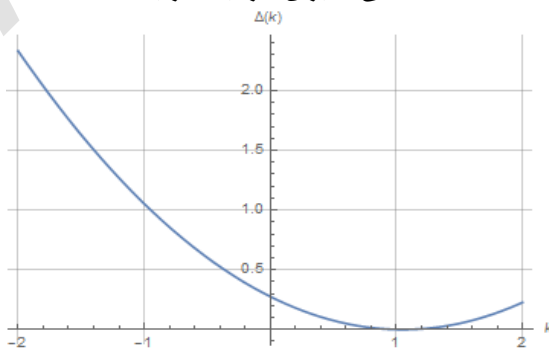
شکل ۳. منحنی k برای تقریب تا مرتبه ۴ مثال ۲
