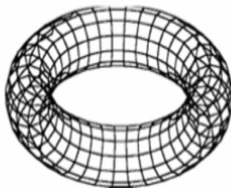
شکل ۴: یک C_4 -نانوچنبره
