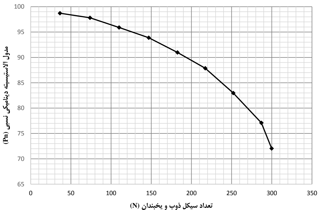
شکل ۸- نمودار تغییرات مدول الاستیسیته دینامیکی نسبی با سیکل‌های یخ زدن و ذوب شدن در نسبت اولی
