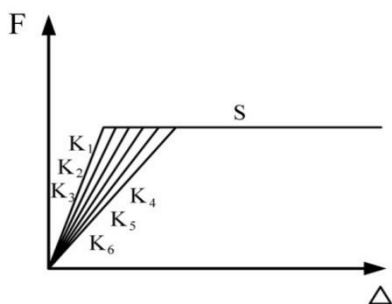
شکل ۴- مقدار سختی متفاوت بر حسب روش‌های محاسبه سختی و مقدار یکتای مقاومت سازه
