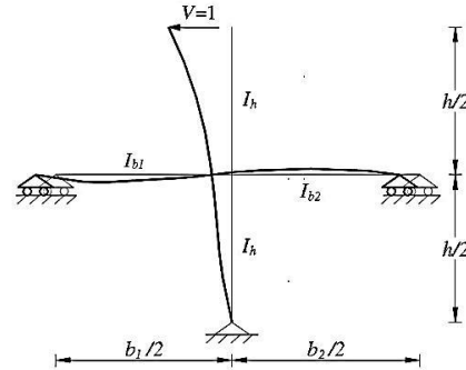
شکل ۷- روش پیشنهادی Heidebrecht and Stafford Smith برای محاسبه سختی [۱۸]
