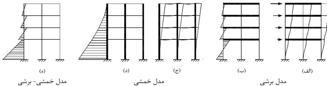
شکل ۶- نحوه تغییر شکل و توزیع ممان در مدل‌های برشی و خمشی؛ (الف) تغییر شکل مدل برشی، (ب) توزیع ممان در مدل برشی، (ج) تغییر شکل مدل خمشی، (د) توزیع ممان در مدل خمشی (ه) توزیع ممان در مدل خمشی - برشی [۶]
