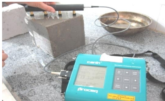
شکل ۱۱- دستگاه سنجش مقاومت الکتریکی و نحوه استفاده از آن
