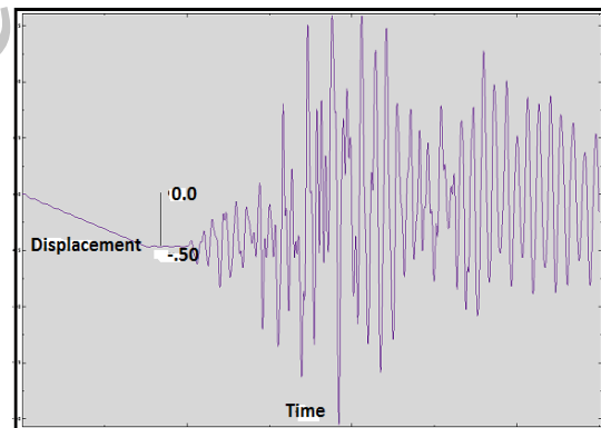
شکل ۴-۵ تاریخچه زمانی جابجایی نسبی تاج سد Koyena
