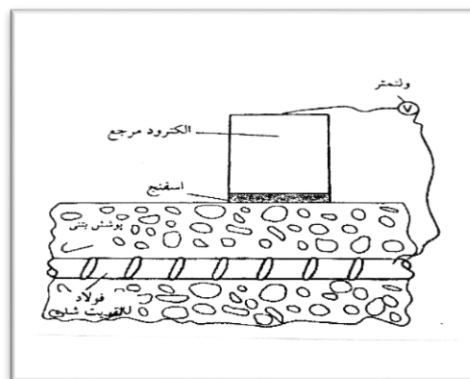
شکل ۴- شکل شماتیک روش نیم پیل
