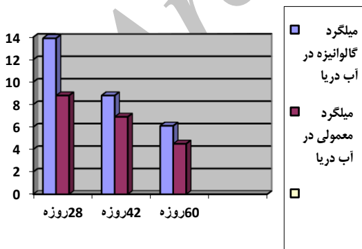
نمودار شماره ۳- نمودار مقایسه‌ای نفوذ یون کلر در نمونه بتنی همراه با میلگرد گالوانیزه و معمولی در مجاورت آب دریا
