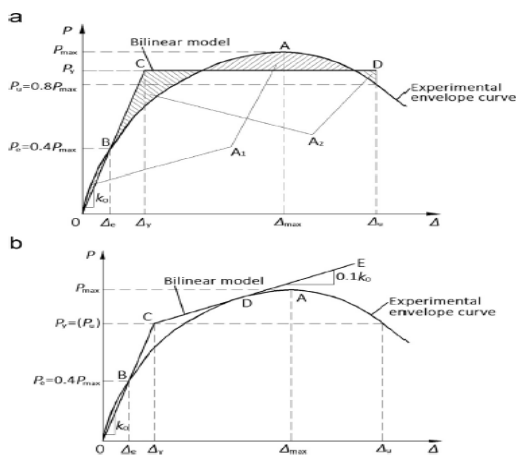
شکل ۱۲- نمایی از تعریف منحنی دوخطی معادل برای ارزیابی شاخص [۲۲]
