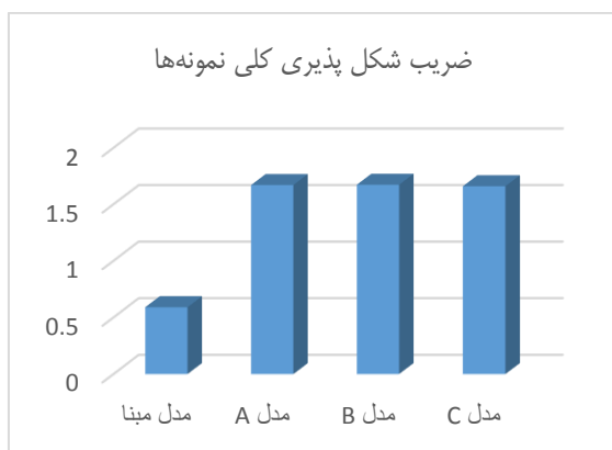
شکل ۱۵- ضریب شکل‌پذیری کلی نمونه‌های
