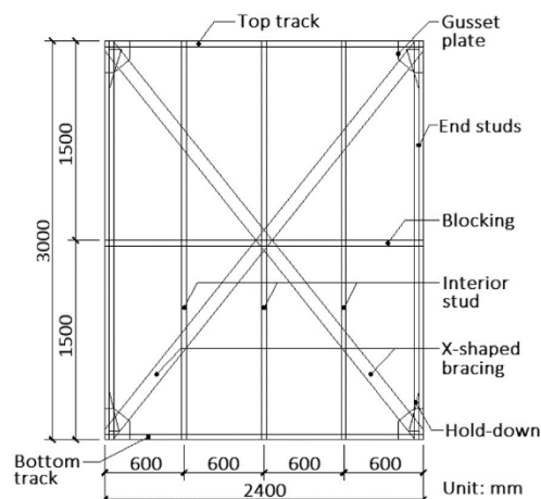
شکل ۴- جزئیات مقاطع [۲۲]
