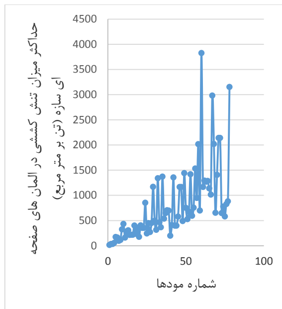
شکل ۱۰- حداکثر تنش بدست آمده کششی در اعضای صفحه ای سازه
