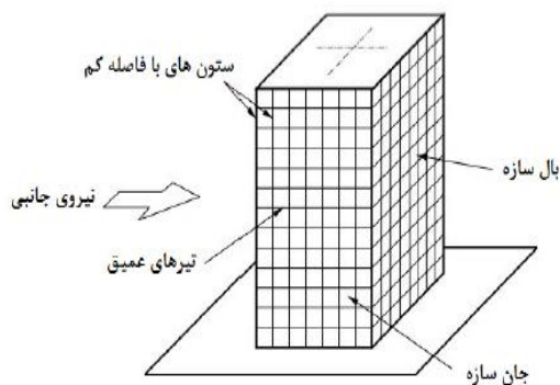
شکل ۳- وضعیت توزیع تنش محوری در ستون‌های بال و جان سازه و وقوع پدیده لنگی برش تحت اثر بار جانبی
