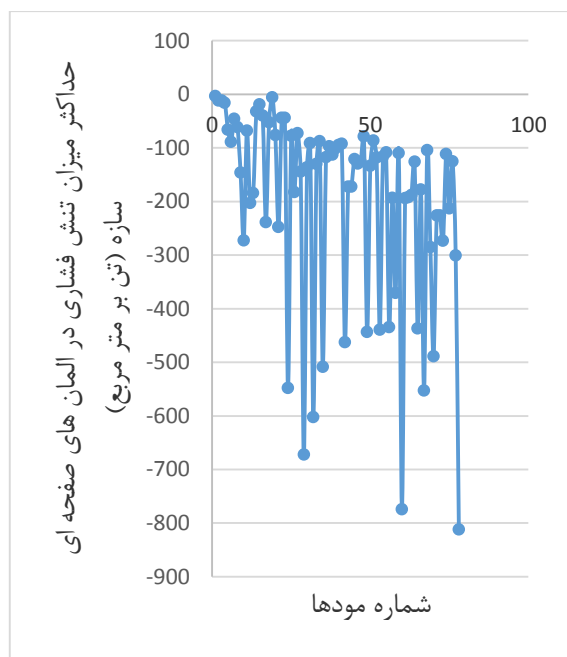
شکل ۱۱- حداکثر تنش بدست آمده فشاری در اعضای صفحه ای سازه
