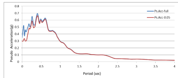
شکل ۱۲- ۲ طیف شبه شتاب برای زلزله اصلی و زلزله تولید شده - اختلاف مقادیر حداکثر ۴,۵٪
