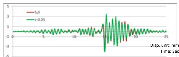
شکل ۱۸- ۱۰ پاسخ تغییر مکان سیستم ۰,۵ ثانیه- اختلاف حداکثر ۶ درصد بیشتر
