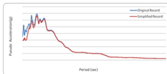
شکل ۱۷- ۹ طیف شبه شتاب برای زلزله اصلی و زلزله تولید شده - اختلاف مقادیر حداکثر ۴٪
