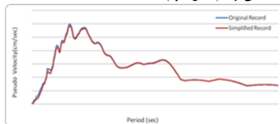
شکل ۱۶- ۸ طیف شبه سرعت برای زلزله اصلی و زلزله تولید شده - اختلاف مقادیر حداکثر ۲٪
