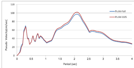
شکل ۱۴- ۱ مقایسه طیف شبه سرعت برای زلزله اصلی و زلزله تولید شده - اختلاف مقادیر حداکثر ۵٪
