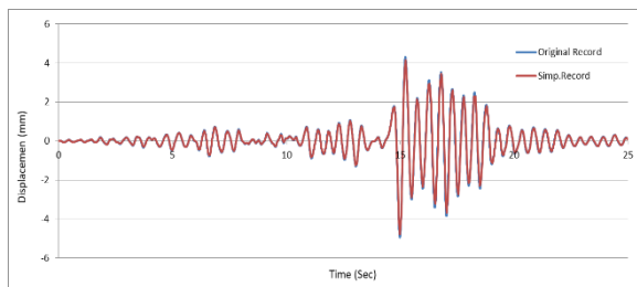
شکل ۱۶-۱ پاسخ تغییر مکان سیستم ۲ درجه آزاد ۰,۵ ثانیه- اختلاف مقادیر حداکثر ۳٪
