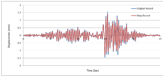
شکل ۱۵-۱ پاسخ تغییر مکان سیستم ۲ درجه آزاد ۰,۳ ثانیه- اختلاف مقادیر حداکثر ۱۱٪
