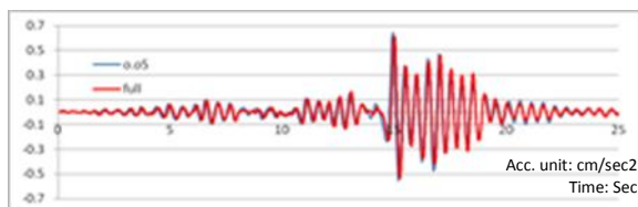
شکل ۱۰- ۲ پاسخ شتاب سیستم ۰,۵ ثانیه- اختلاف حداکثر ۶ درصد بیشتر
