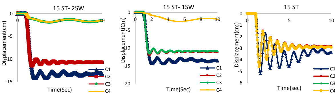
شکل ۳۸- جابجایی عمودی محل حذف ستون‌ها در قاب 15ST2SW
