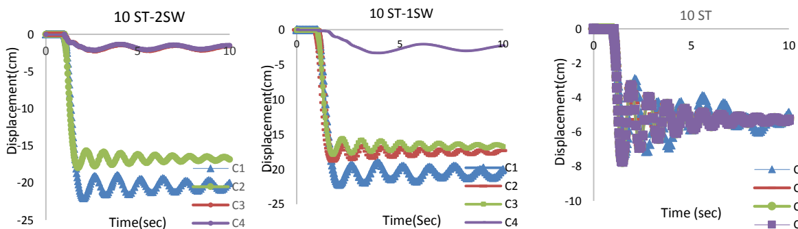
شکل ۳۵- جابجایی عمودی محل حذف ستون‌ها در قاب 10ST2SW
