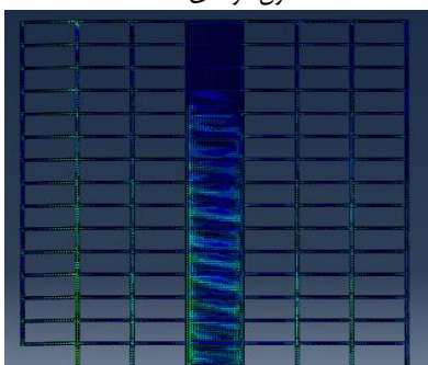
شکل ۵۶- تحلیل قاب 15ST1SW با حذف ستون گوشه‌ی C1
