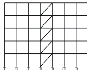
شکل ۱۳- قاب فولادی ۵ طبقه دارای سیستم دوگانه
