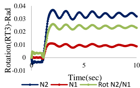
شکل ۴۸- دوران مفصل پلاستیک تیرهای مجاور محل حذف ستون C 1 در قاب 10ST1SW
