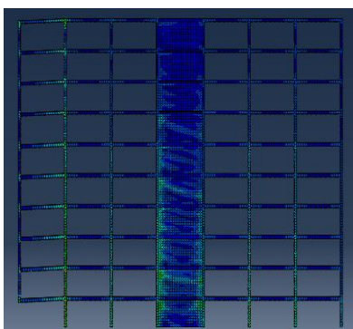
شکل ۵۳- تحلیل قاب 10ST1SW با حذف ستون گوشه‌ی C1
