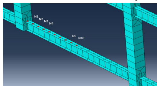
شکل ۳۹- تعریف گره‌های مرجع جهت محاسبه دوران گره‌های مختلف در طول تیرها
