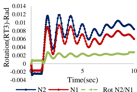
شکل ۴۹- دوران مفصل پلاستیک تیرهای مجاور محل حذف ستون C 1 در قاب 10ST10ST1SW
