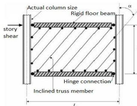
شکل ۱۹- مدل نواری در طراحی دیوار برشی فولادی [۱۷]
