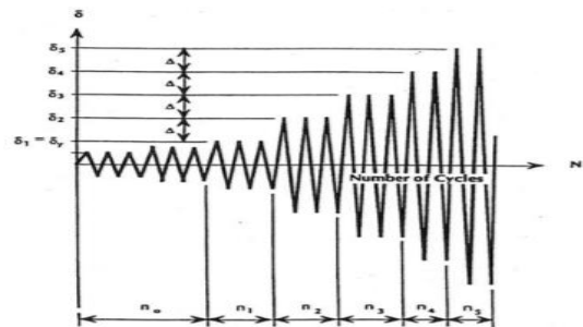
شکل ۳- پروتکل بارگذاری چرخه‌ای مطابق استاندارد ATC-24 [۱۴] مطابق شکل (۴)، بار چرخه‌ای به بالای مدل اجزا محدودی دیوار برشی فولادی اعمال شده است.
